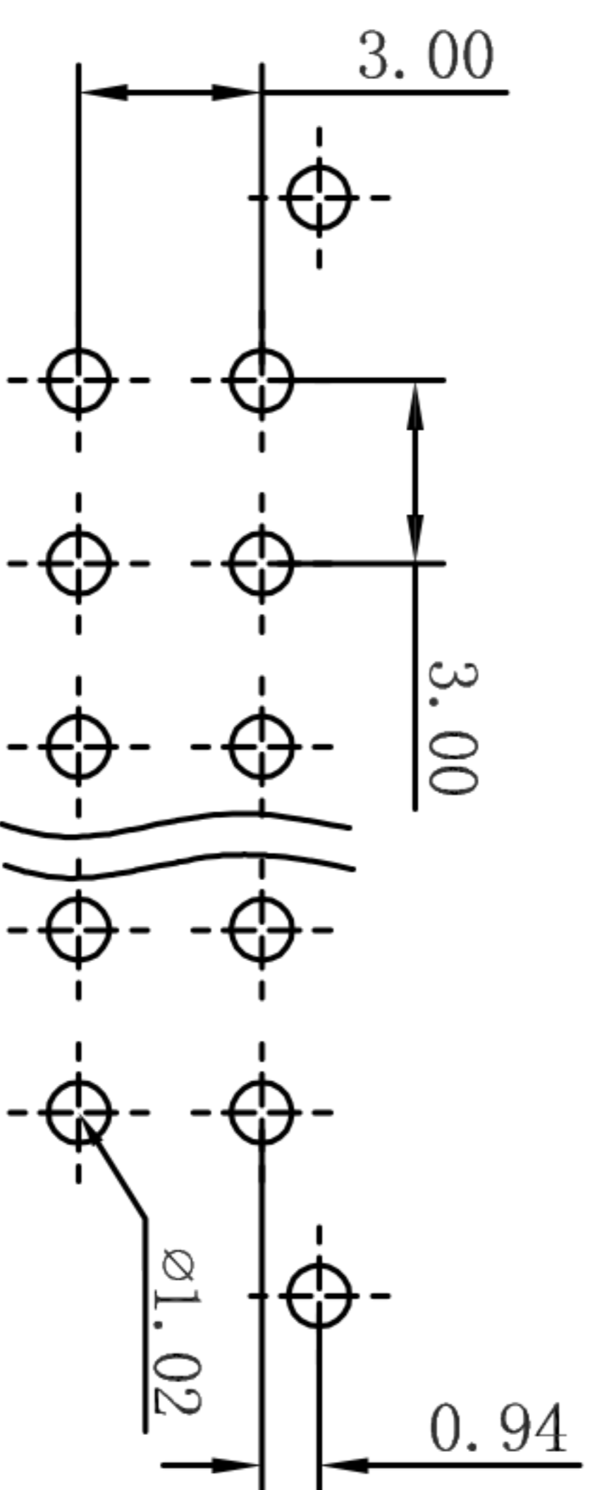
P.C.B. LAYOUT
